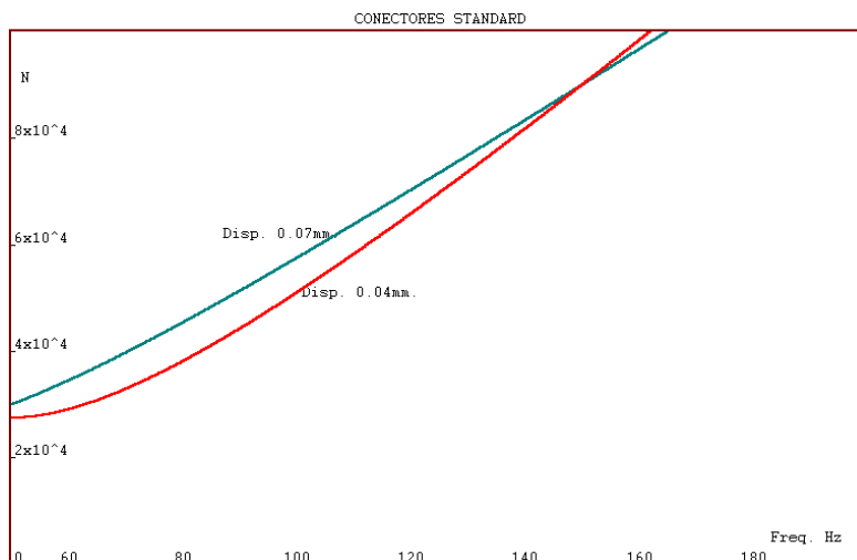
Fig. N° 12: Deflexiones admisibles en función de la frecuencia y n° de ciclos
