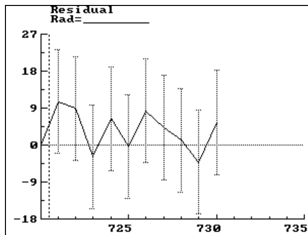
Fig.7 : Comportamiento residual en las predicciones de radiación (eje x en días)
