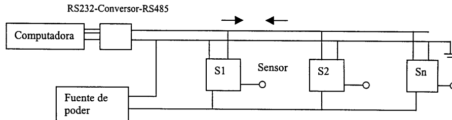
Figura 1. Esquema de un sistema de adquisición con conexión seriada
