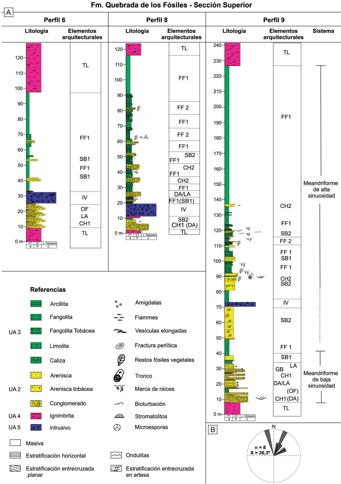
Figura 10. a) Perfiles sedimentológicos de la sección superior de la Formación Quebrada de los Fósiles. b) Diagrama de rosas que muestra las paleocorrientes medidas. Figure 10. a) Sedimentological sections of the upper section of the Quebrada de los Fósiles Formation. b) Rose diagram showing the paleocurrent readings.
