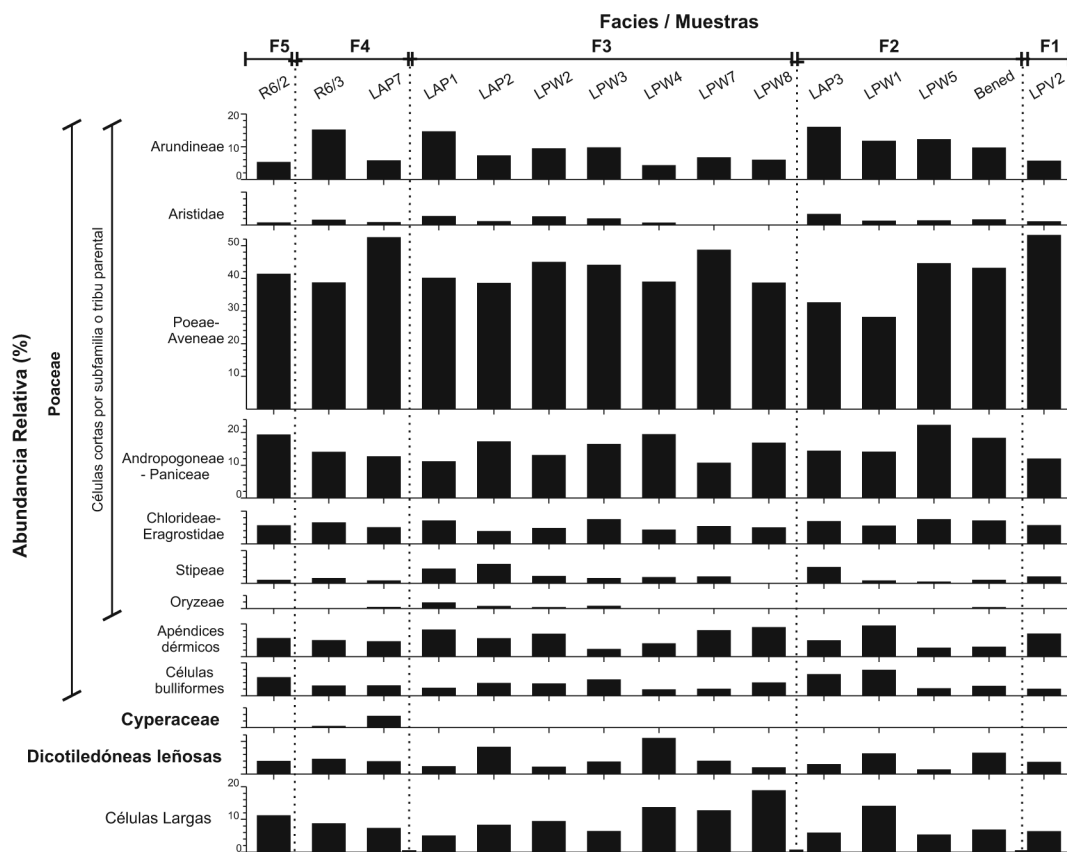
Figura 3. Contenido de fitolitos en las muestras de las diferentes facies del Pleistoceno tardío. Figure 3. Phytolith content from samples of different recognized late Pleistocene facies.
