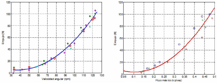
Figura 6. Izquierda: Velocidad Angular (RPM) vs Empuje (N).
