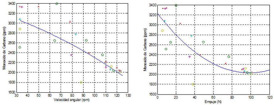
Figura 7. Izquierda: Velocidad Angular (RPM) vs Monóxido de carbono (ppm).
