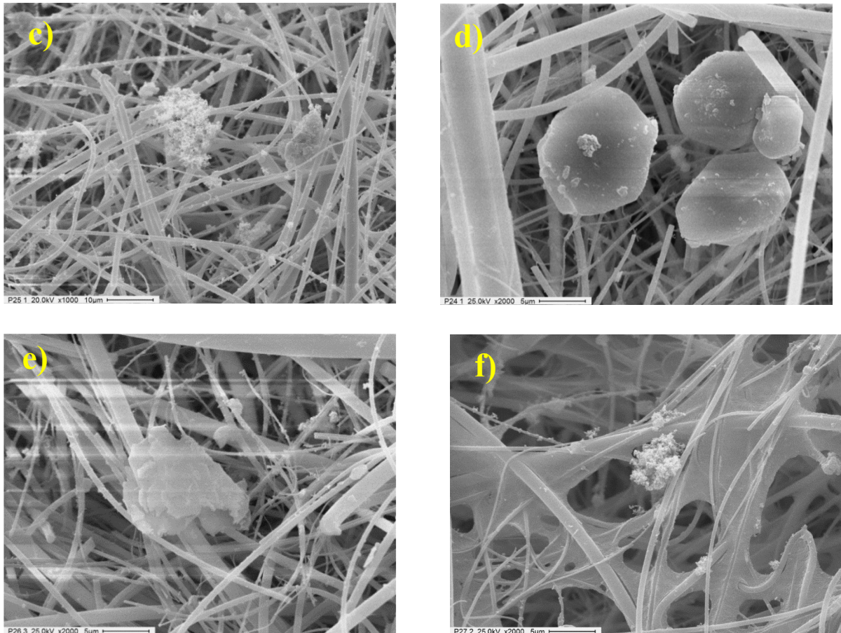
Figura 5. Micrografías de partículas de las zonas industrial a) y b), urbana c) y d) y residencial e) y f)
