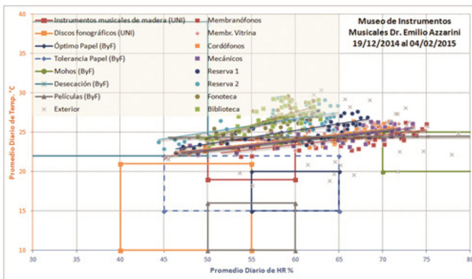
Gráfico 1. Promedio Diario Temp y HR. Verano 2014/2015 (García Santa Cruz, M. G. 2016)
