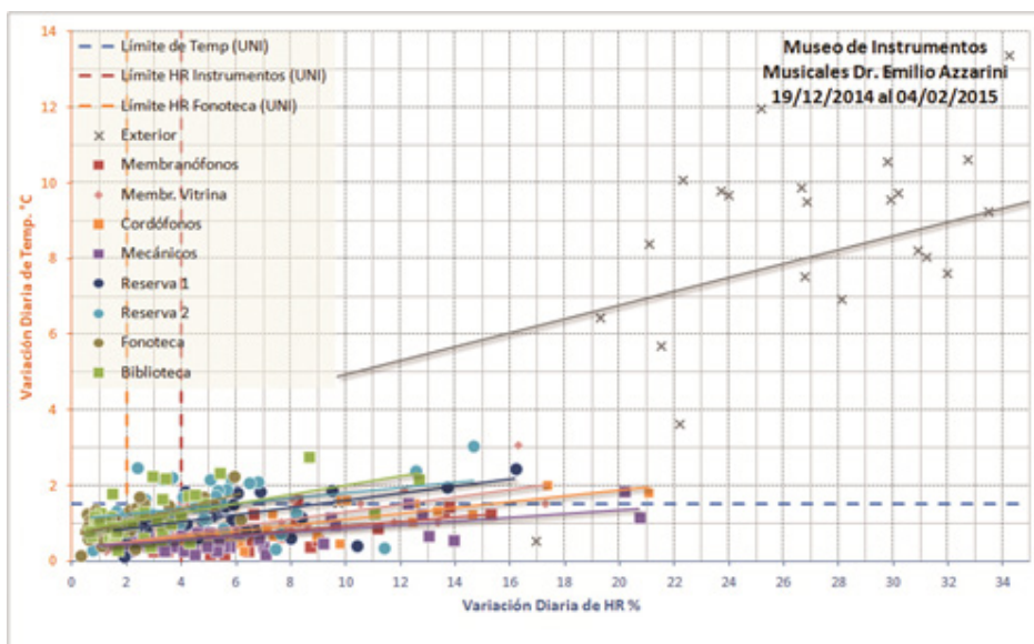
Gráfico 2. Variación Diaria de Temp HR. Verano 2014/2015 (García Santa Cruz, M. G. 2016)
