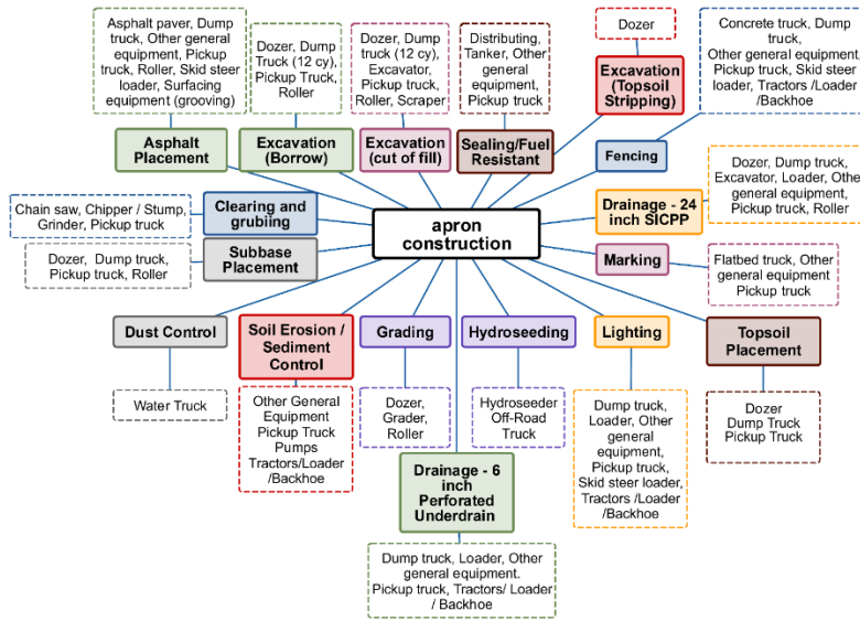
Figura 4. Construcción de plataforma: actividades y equipamiento por actividad, elaboración propia basada en [3]
