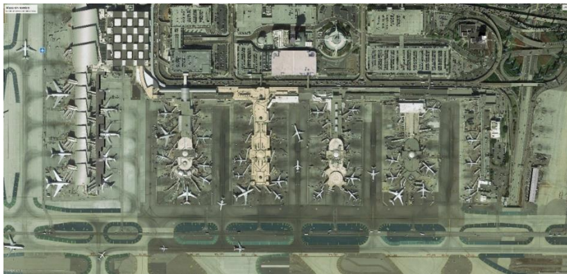
Figura 5. Concepto Espigón: Aeropuerto Internacional de Los Ángeles.
