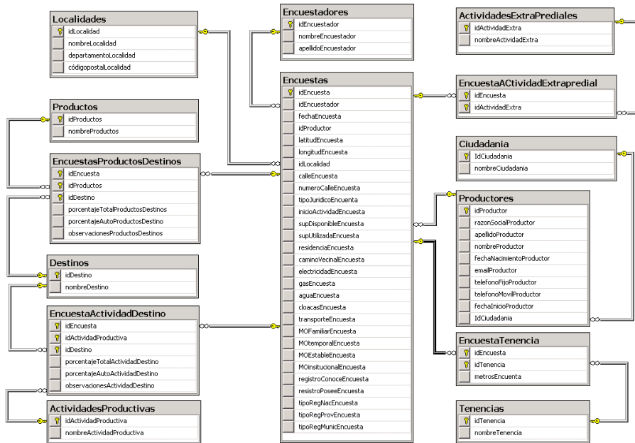
Fig. 3. Diagrama de Entidad Relación
