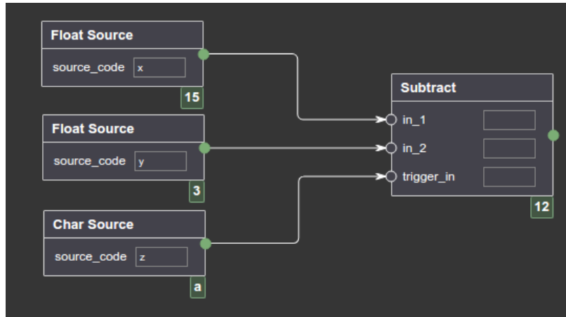
Figura 46:: Ejemplo de ejecución condicional: estado #4
