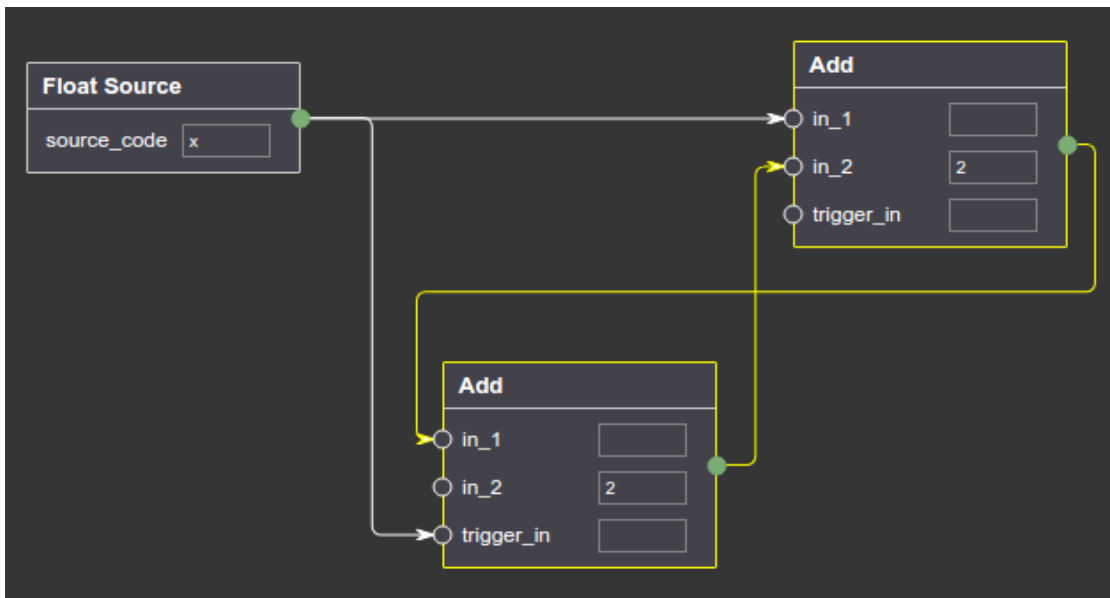
Figura 50: Conversión de ciclo crítico en no crítico
