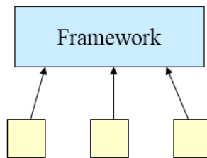
Figura 19: Framework instanciado
