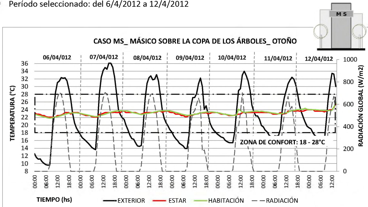
Figura IV.23. Temperatura exterior e interiores en otoño de la vivienda másica sobre la copa
