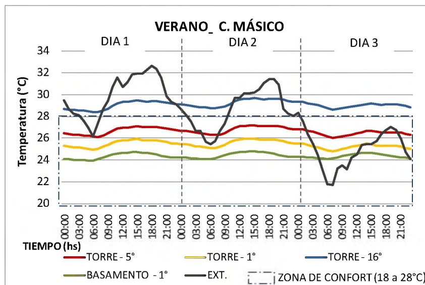
Figura V.26. Comportamientos térmicos de verano en unidades de vivienda a diferentes alturas en edificios mássicos
