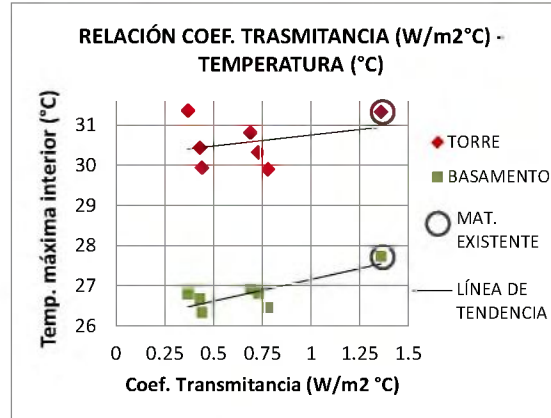
Figura VI.2. Relación de coeficientes de trasmittancia en la envolvente y temperaturas
