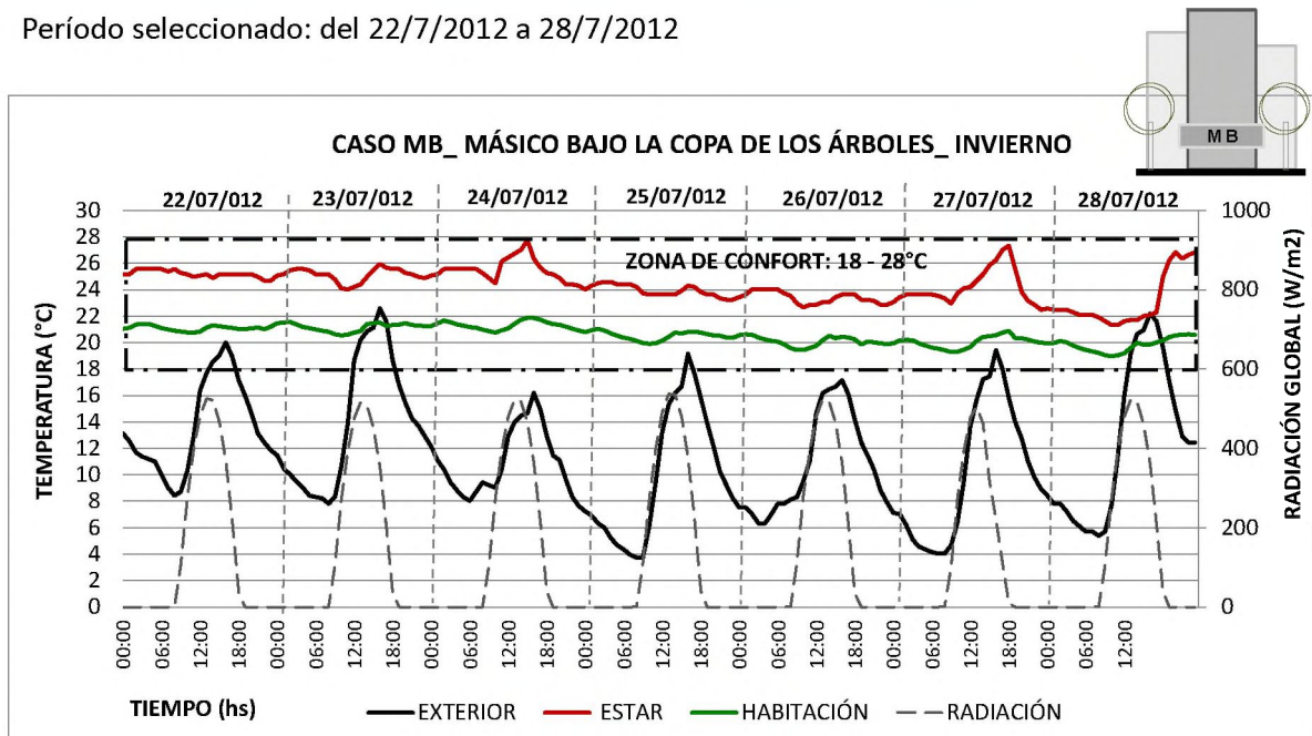
Figura IV.19. Temperatura exterior e interiores en invierno de la vivienda másica bajo la copa
