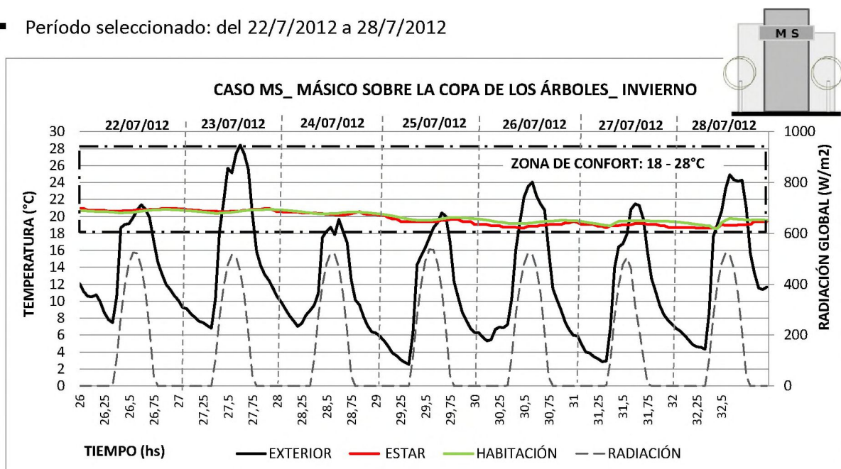
Figura IV.24. Temperatura exterior e interiores en invierno de la vivienda másica sobre la copa
