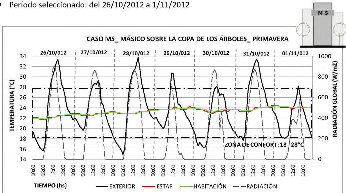
Figura IV.25. Temperatura exterior e interiores en primavera de la vivienda másica sobre la copa
