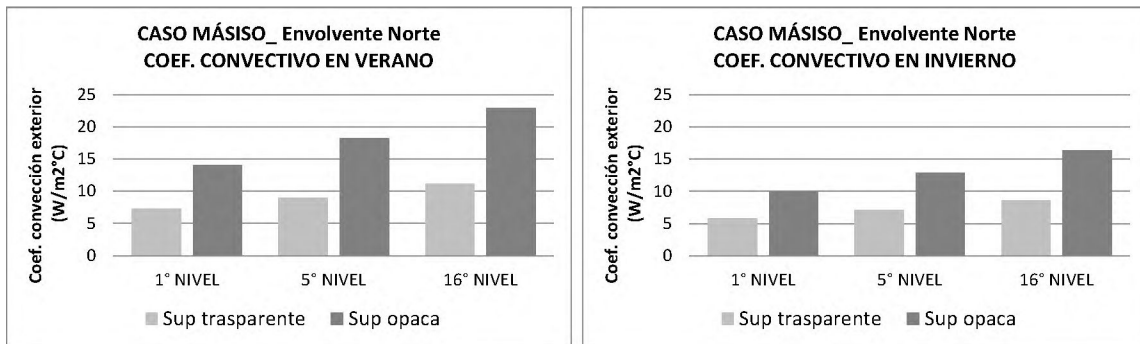
Figura V.24. Coeficientes convectivos para superficies expuestas al Norte en edificios másicos
