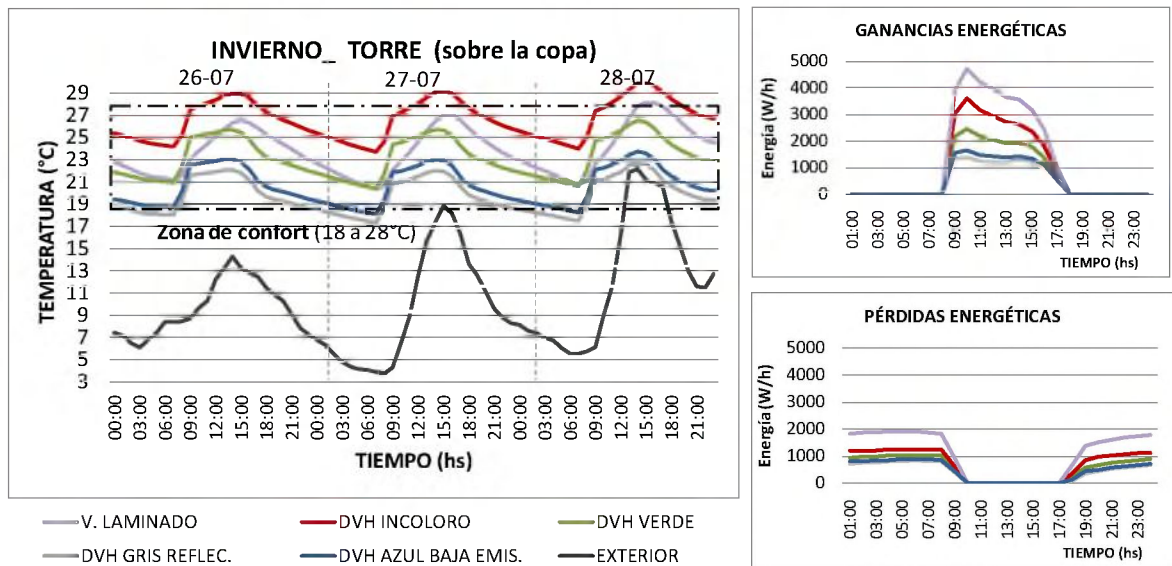
Figura V.18. Temperaturas interiores y ganancias y pérdidas energéticas de los vidrios evaluados en invierno en la Torre
