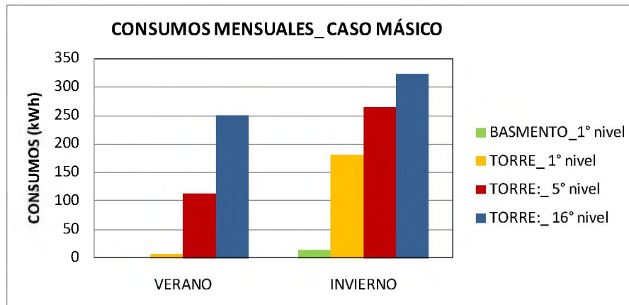
Figura V.28. Consumos mensuales para climatización en unidades de vivienda a diferentes alturas en edificios másicos
