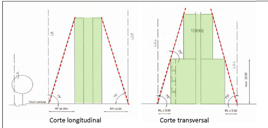
Figura III.16. Tipología edilicia en torre con retiros y alturas mínimas según limitación de ángulos
