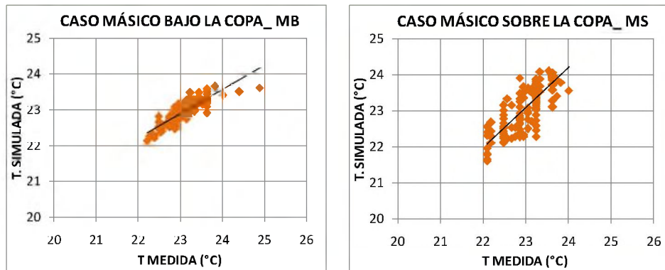
Figura V.5. Correlación temperatura medida y simulada de las dos viviendas del caso másico
