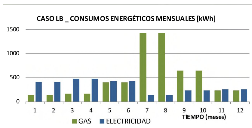
Figura IV.34. Consumos mensuales de la vivienda liviana bajo la copa de los árboles
