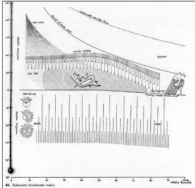
Figura II.13. Gráfico esquemático de la zona de confort de Olgay (Olgay, 1963)
