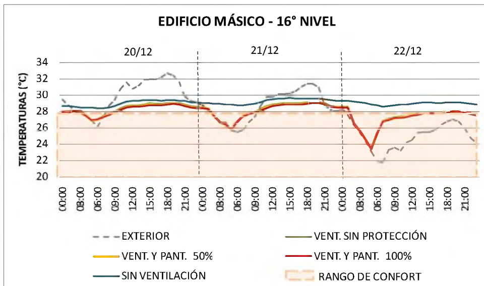
Figura V.37. Comportamiento térmico mediante la aplicación de ventilación natural y protecciones verticales en el nivel superior del caso másico
