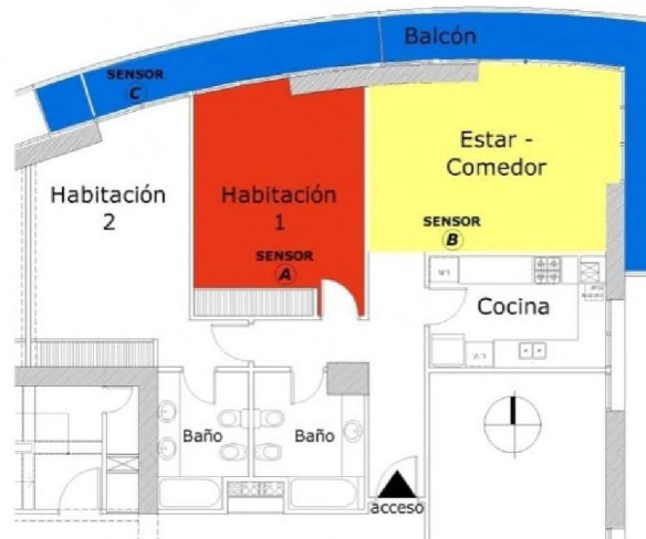
Figura IV.27. Planta de la vivienda liviana
