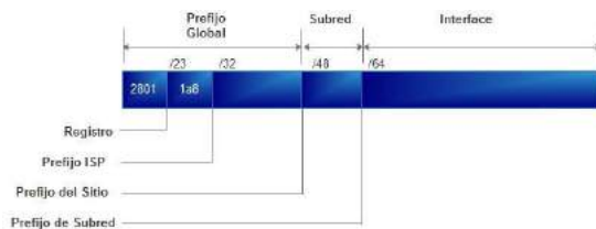
Figura 3: Máscaras IPv6
