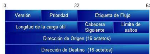
Figura 2: Cabecera IPv6
