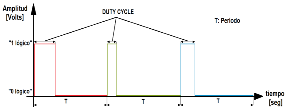
Fig. 5. Ejemplo de modulación por ancho de pulso (PWM)
