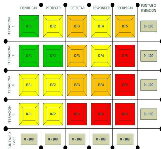
Fig. 4. Interfaz de explotación del Framework propuesta
