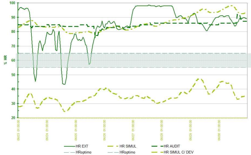
Figura 8: Humedad relativa en el transcurso del período estudiado para datos exteriores, de auditoría, simulados en las condiciones actuales y simulados con DEV.
