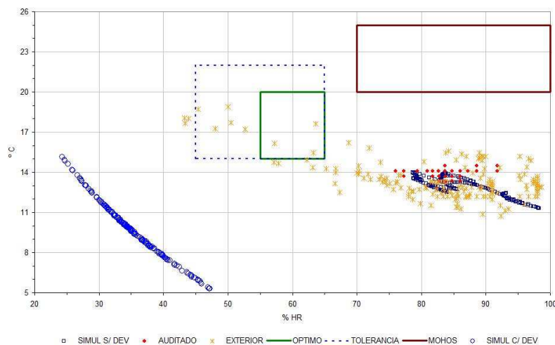
Figura 11: Comparación de los datos exteriores, auditados y simulados con las condiciones óptimas de conservación de Bell y Faye.
