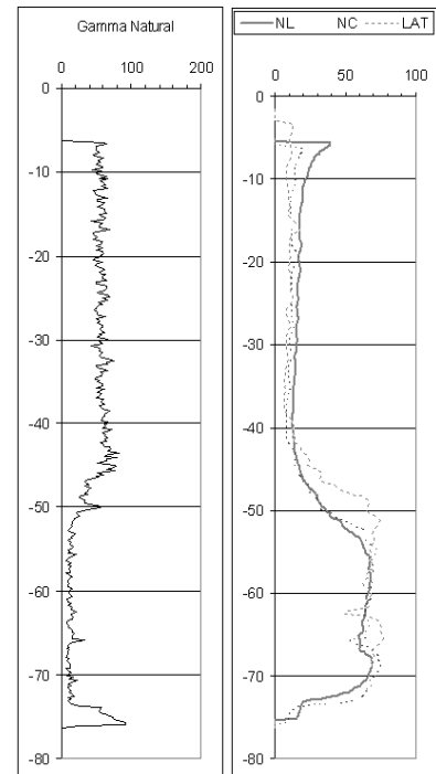
Figura 2. Perfilaje geofísico.
