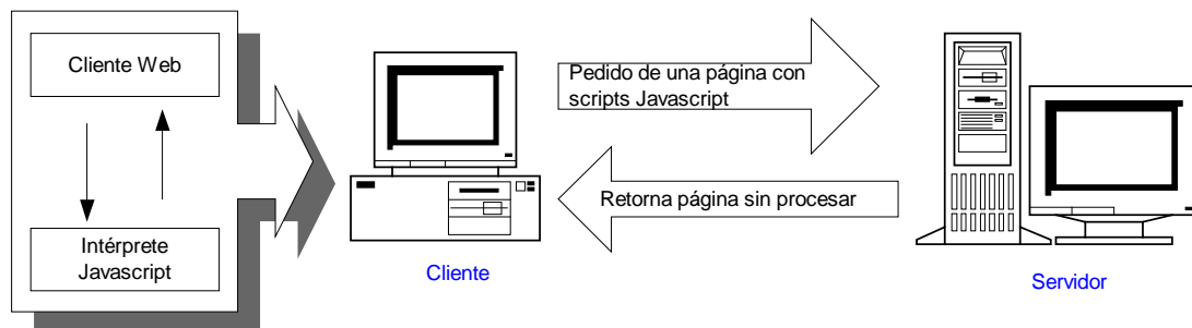
Fig. 2: El cliente web solicita una página que contiene uno o más scripts Javascript. Cuando el servidor web se encuentra con este requerimiento simplemente la retorna como cualquier otra página y la ejecución de los scripts se realiza en el cliente antes de visualizar la página al usuario final.
