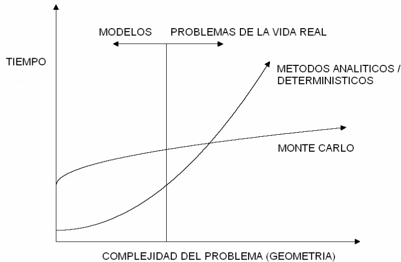
Fig. 1: Métodos determinísticos vs. Monte Carlo
