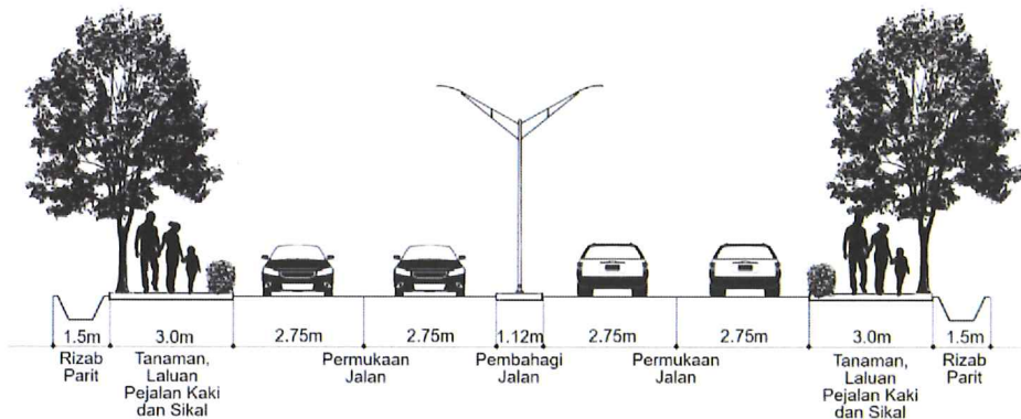
Rajah 4: Keratan Rentas Rizab Jalan Pengumpul Kecil Empat Lorong Dua Hala (20.12 meter / 66.01 kaki).
