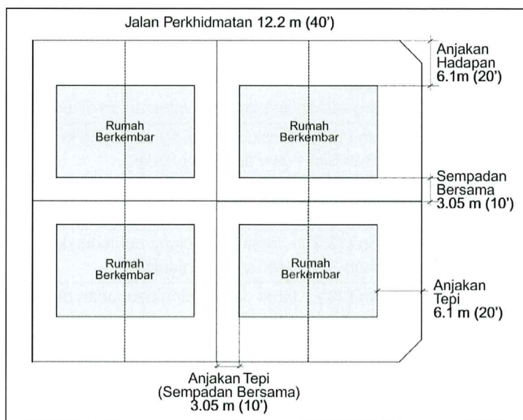
Rajah 17: Lakaran Anjakan Bangunan Rumah Berkembar.
