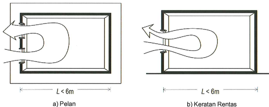
Rajah 25: Kedalaman Efektif ( L ) Bilik untuk Pengudaraan Satu Sisi.
