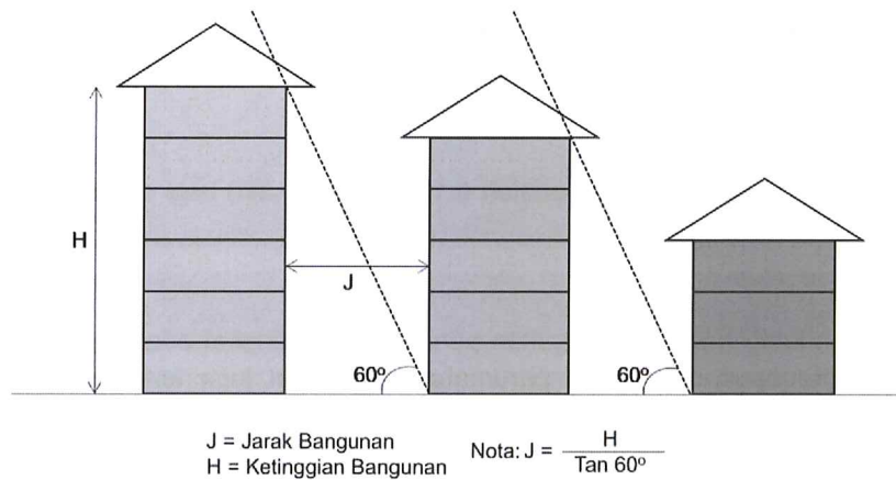
Rajah 20: Ilustrasi Piawaian Anjakan Antara Bangunan Tidak Sama Tinggi Bagi Pembangunan Perumahan Berbilang Tingkat
