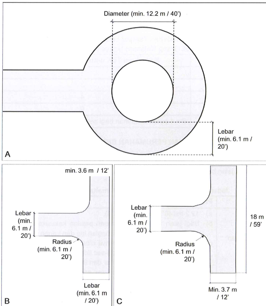
Rajah 14: Jenis Reka Bentuk Cul-de-Sac .
