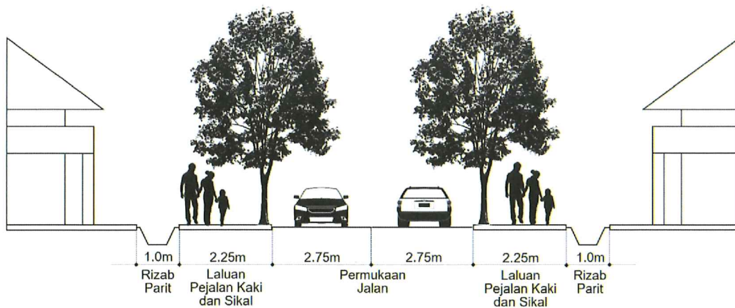
Rajah 13: Keratan Rentas Rizab Jalan Tempatan Dua Lorong Dua Hala (12 meter / 40 kaki).
