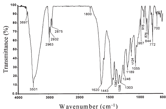
FIG. 2. IR spectrum of solid gossypol.
