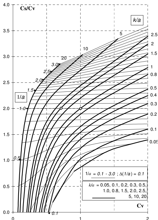
Slika 1. Zavisnost odnosa C_S/C_V od koeficijenta varijacije C_V za troparametarsku gama raspodelu.
