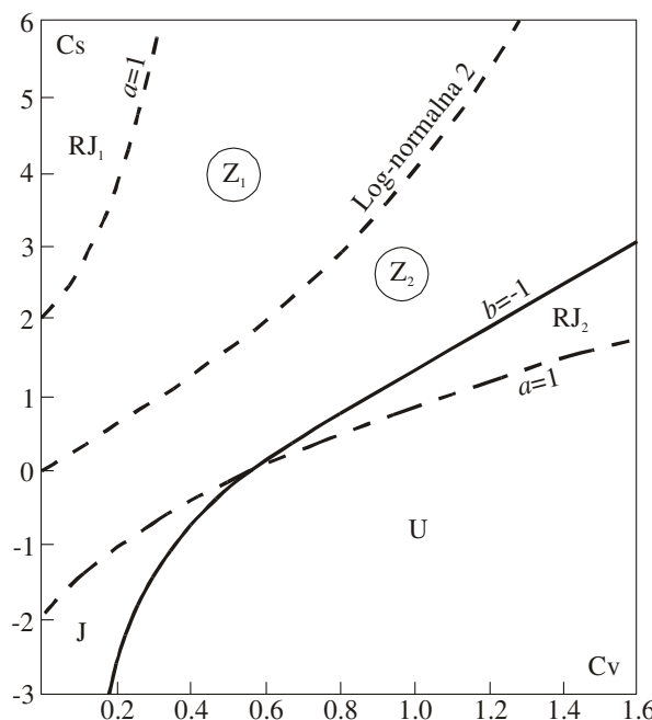
Slika 3. Oblasti različitih oblika gustine logaritamske Pearson III raspodele.
