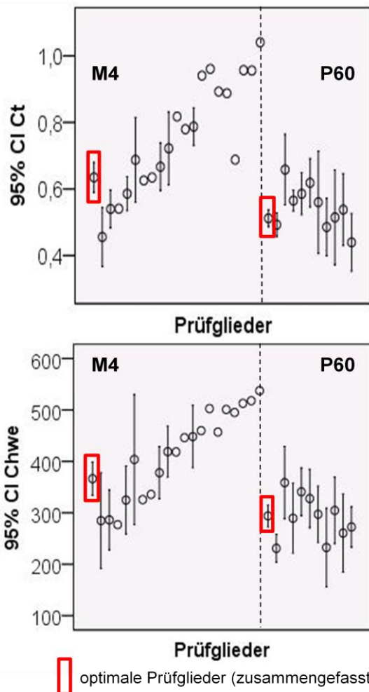
Abb. 2: 95% CI der Mittelwerte der C_{org} - und C_{hwe} -Gehalte der optimalen und suboptimalen Prüfglieder im M4 und P60
