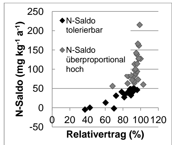
Abb. 1: Beziehung zwischen N-Saldo und Relativertrag (% des mittleren Maximalertrages) in den Versuchen P60 und M4. ( N_{Saldo} = N_{Düngung} + N_{sonstige\ Quellen} - N_{Entzug} )
