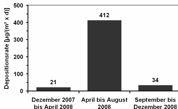
Abbildung 1: Phosphor-Deposition nach Jahresabschnitten
