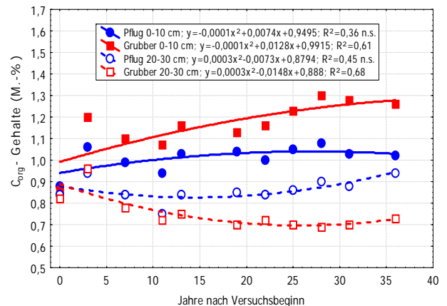
Abb.1: Veränderung der tiefenabhängigen TOC-Gehalte bei verschiedener Bodenbearbeitung (Seehausen, Versuch 1)
