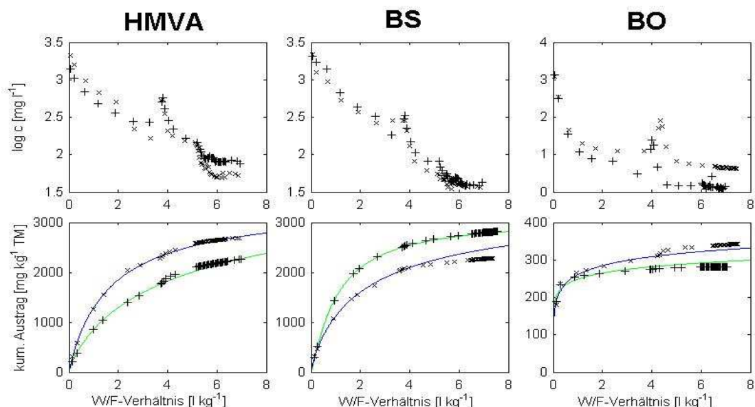
Abb. 2: Ergebnisse der Säulenversuche für das Element Kupfer.
