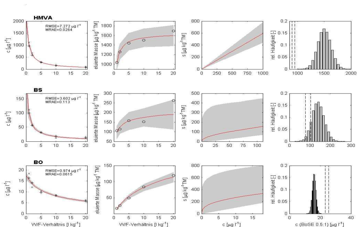
Abb. 1: Ergebnisse der Schüttelversuche für das Element Kupfer.
