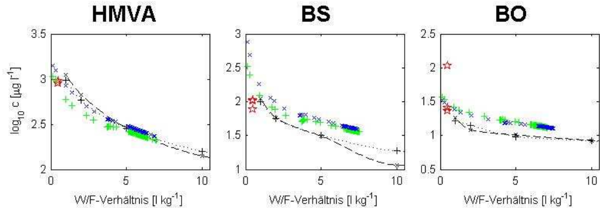
Abb. 3: Vergleich zwischen den verschiedenen Säulen- und Schüttelversuchen für das Element Kupfer.
