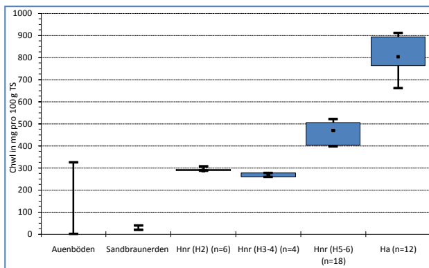
Abbildung 3: C hwl – Werte von Auenböden (Rinklebe et al., 2001) und Oberböden von Sandbraunerden (Landgraf, 2001) im Vergleich zu verschiedenen Torfen (Hnr= Radizellentorf; Ha= amorpher Torf; in Klammern der jeweilige Humositätsgrad (H))
