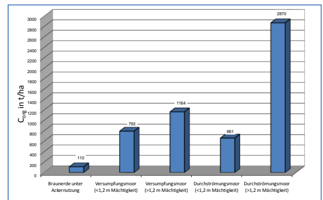
Abbildung 2: Vergleich der Kohlenstoffspeichermenge eines Mineralbodens mit verschiedenen Moorböden (Quelle für die Braunerde: Leifeld et al., 2003)
