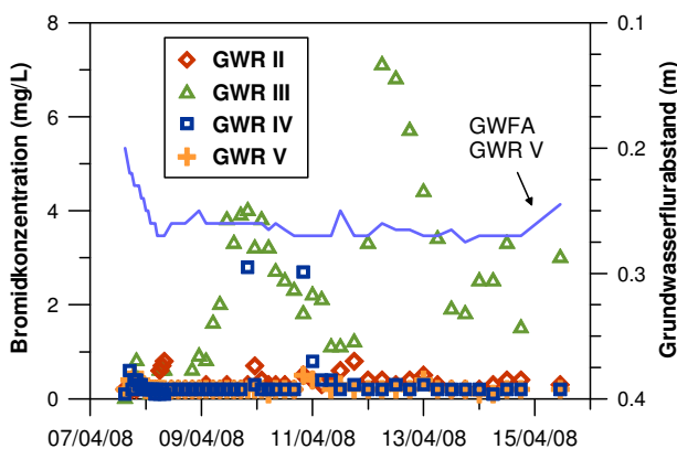
Abbildung 5: Bromidkonzentrationen der Grundwasserrohre GWR II-V und Grundwasserflurabstand am GWR V.
