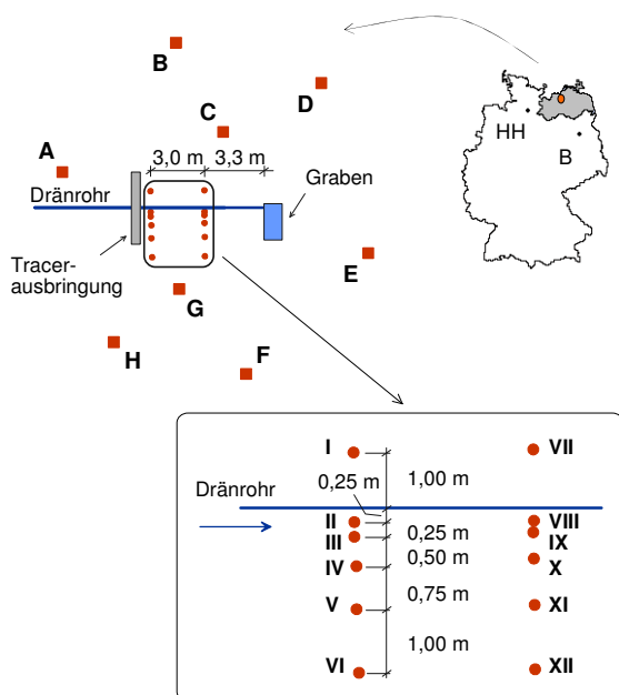
Abbildung 1: Versuchsaufbau
