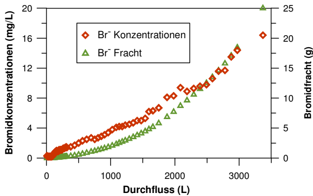
Abbildung 4: Bromidkonzentrationen und -frachten am Dränrohr. Versuchsende nach ca. 3400 L bzw. 8 Tagen.
