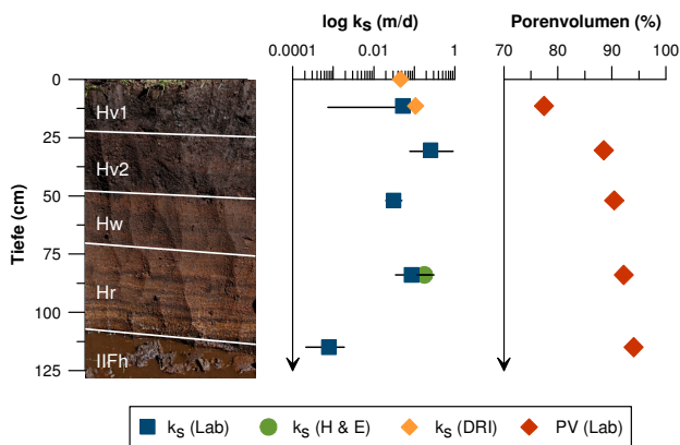
Abbildung 2: Ausgewählte Profileigenschaften: k_s -Werte nach Laborversuchen (Lab), Hooghoudt & Ernst (H & E) und Doppelringinfiltration (DRI) sowie das Porenvolumen (PV).
