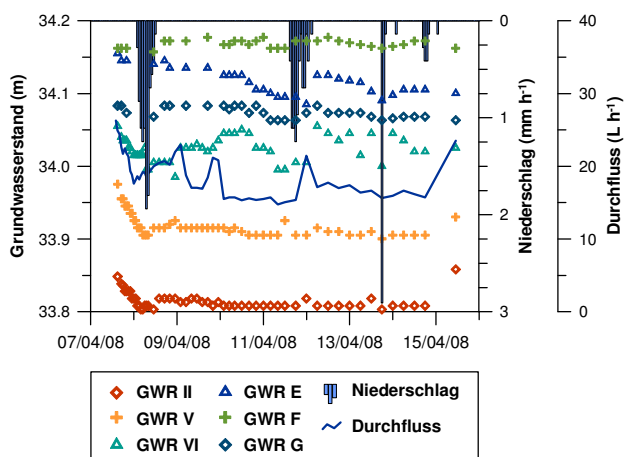
Abbildung 3: Niederschlag, ausgewählte Grundwasserstände und Drändurchfluss.
