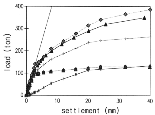
Fig. 15. Pile No. 7.
