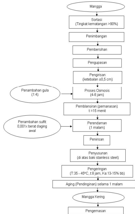
Gambar 1. Diagram Alir Proses Pembuatan Manisan Mangga Kering,
