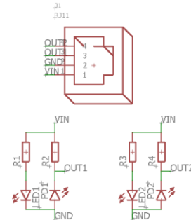
Gambar 4.1 Rangkaian Skematik Sensor Photodioda
