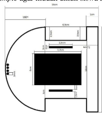
Gambar 4.3 Skematik Robot
