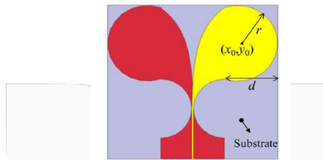
Gambar 1 .Bentuk konfigurasi Antena Vivaldi antipodal sirkualr
