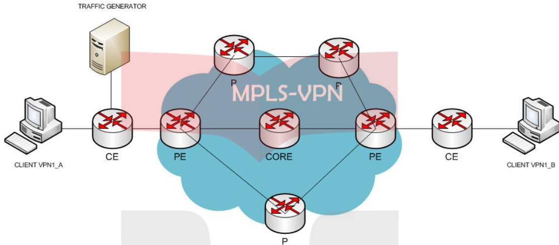
Gambar 1.1 Topologi jaringan
