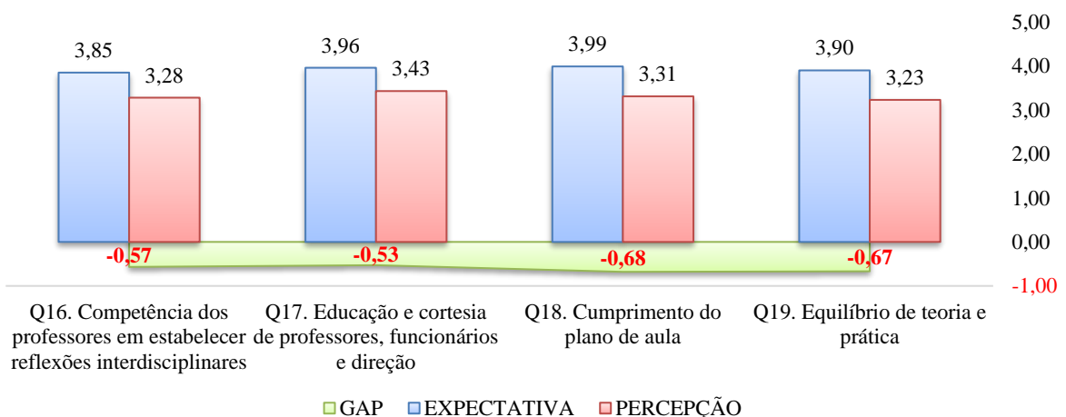
Figura 4 – Dimensão Garantia
