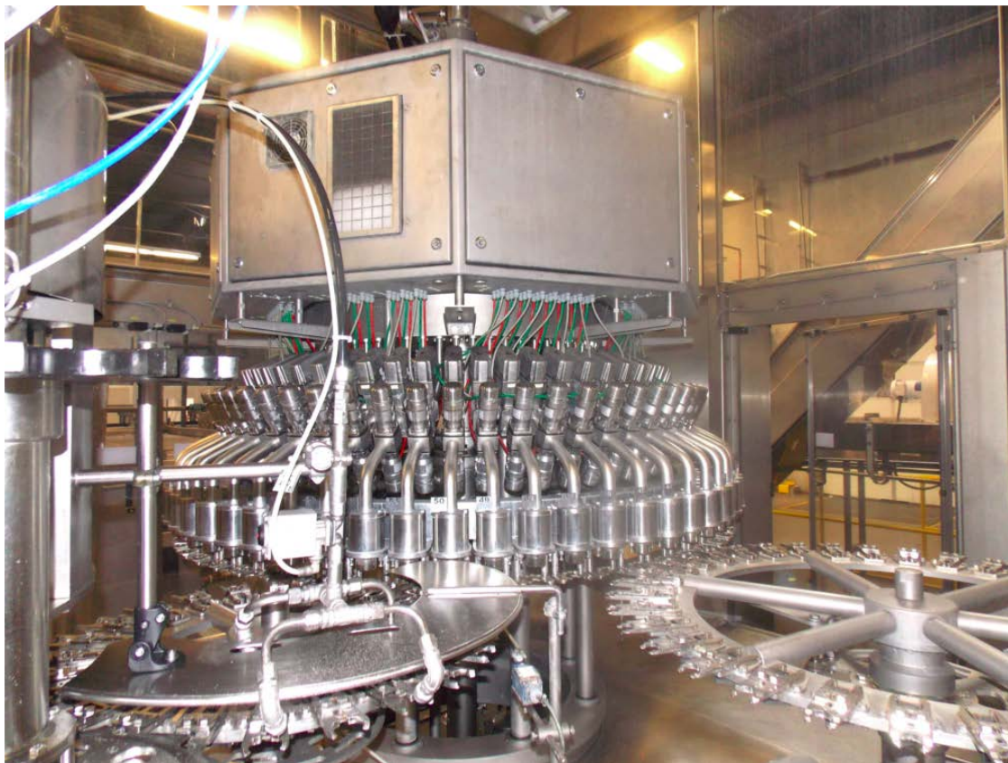
Figura 3: Llenadora Krones
