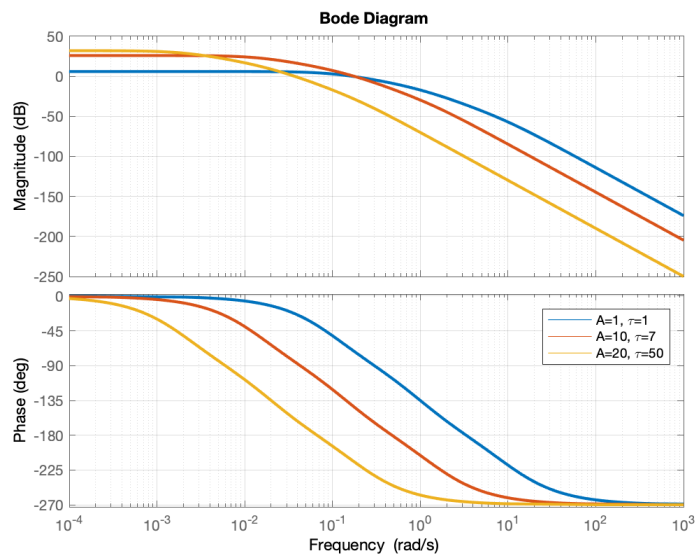
Figura 7: Diagramas de Bode para distintos ejercicios equivalentes, obtenidos con distintos valores de escalado en amplitud ( A ) y frecuencia ( \tau ).
