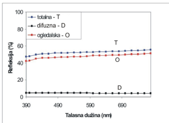
Slika 5 - Krive zavisnosti refleksije svetla od talasne dužine za elektrohemijski uglučane uzorke čelika. Vreme glačanja: a) 2 min i b) 5 min
