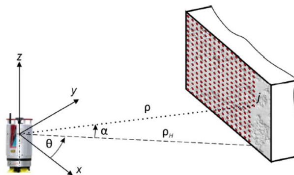
Слика 1 - Принцип скенирања и резултати мерења код ТЛС методе [1]
