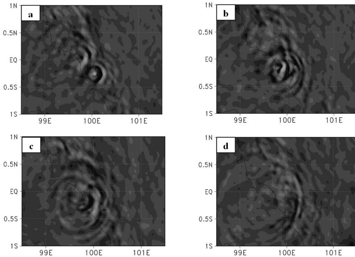
Gambar 3-7: Penampang melintang horizontal kecepatan angin vertikal ( \text{m s}^{-1} ) hasil model domain 3 yang menggunakan skema MRF pada (a) 09:20 UTC, (b) 09:50 UTC, (c) 10:20 UTC, dan (d) 11:00 UTC di ketinggian 19 km
