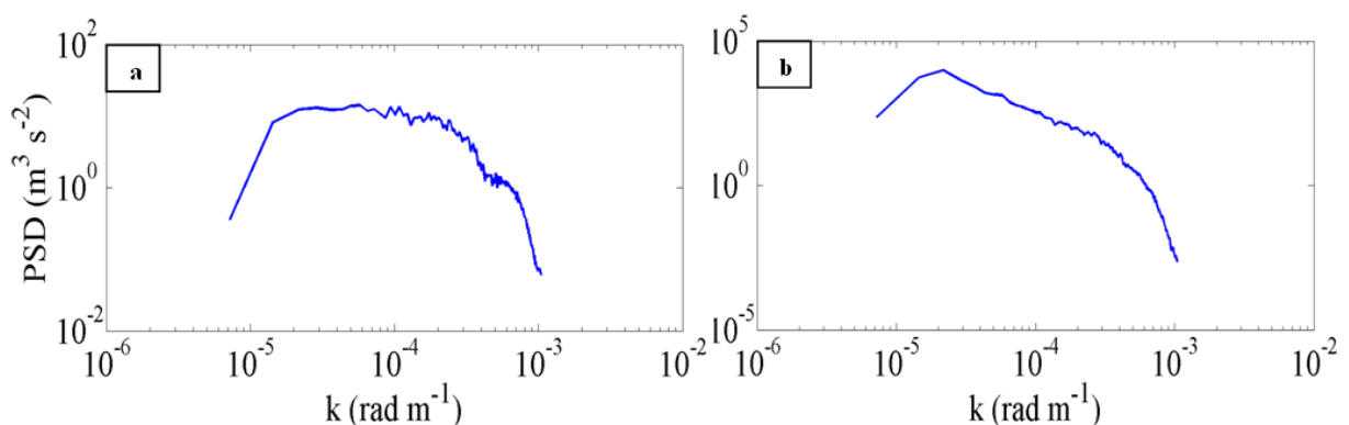
Gambar 3-6: Power Spectral Density kecepatan (a) angin vertikal dan (b) angin horizontal skema MRF terhadap bilangan gelombang pada ketinggian 15 km sepanjang 0,2 \text{ }^{\circ}\text{LS} dari jam ke-3 hingga jam ke-49 simulasi.
