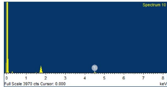
Gambar 5. Hasil pemeriksaan spektrum komposisi kimia Ti-12Cr setelah perendaman dalam larutan NaCl 3% menggunakan EDX.
