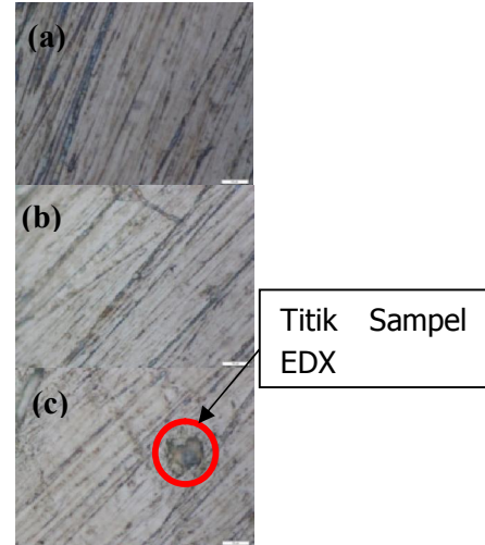
Gambar 4. Hasil pemeriksaan Struktur mikro Ti-12Cr dengan Mikroskop Optik (100X perbesaran) pada perendaman (a) 2 minggu, (b) 4 minggu dan (c) 6 minggu dalam larutan NaCl 3%.
