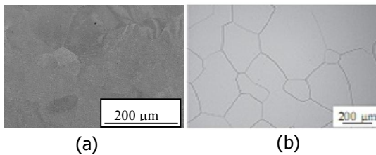
Gambar 2. (a). Hasil SEM paduan Ti-12Cr sebelum diteliti laju korosinya. (b). Hasil Mikroskop Optik paduan Ti-12Cr penelitian terdahulu Liu, dkk (2014).
