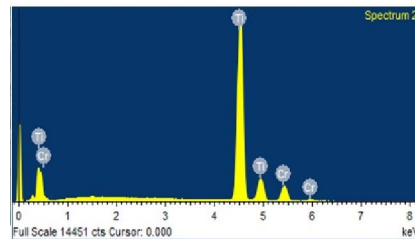
Gambar 3. Spektrum Komposisi kimia Ti-12Cr hasil pemeriksaan SEM-EDX.
