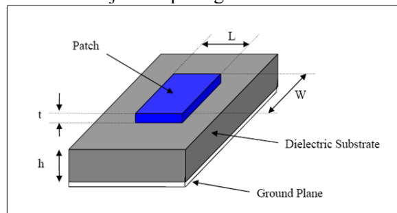
Gambar 2. Susunan Elemen Antena Mikrostrip[2]
