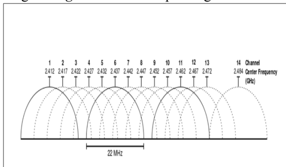
Gambar 1. Pembagian Kanal 2,4 GHz [11]
