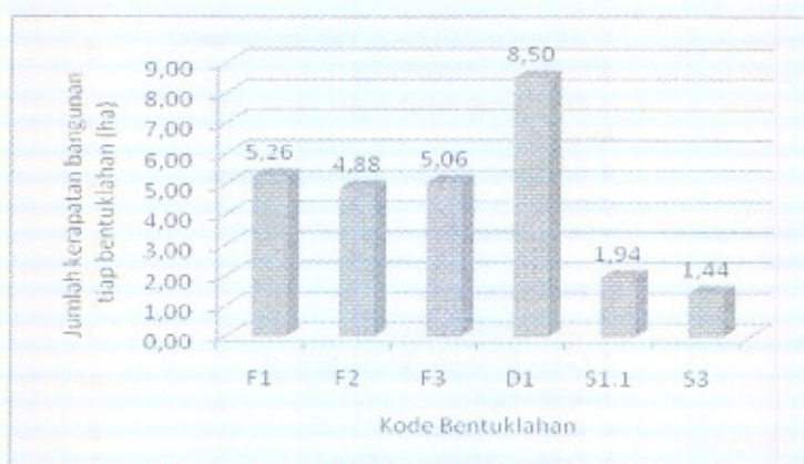
Gambar 3.1 Kerapatan bangunan di enam bentuklahan (Pengolahan data, 2012)
