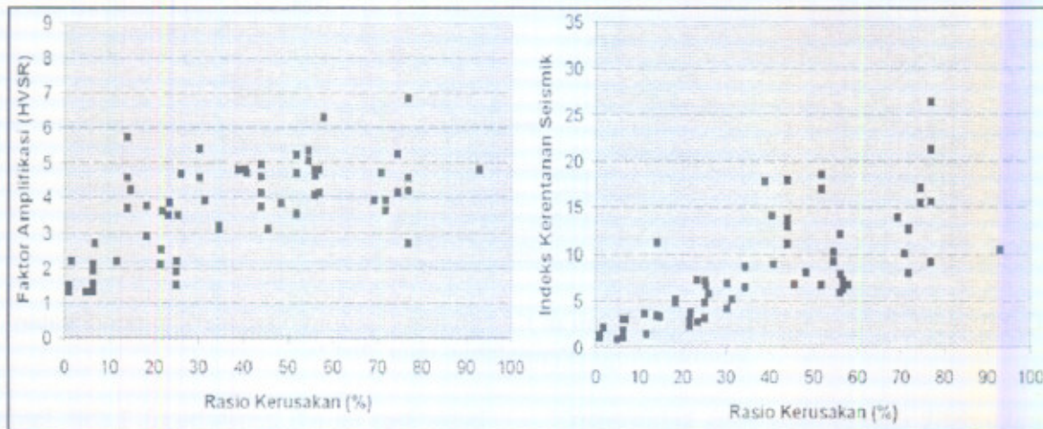
Gambar 3.4 Perbandingan antara faktor amplifikasi dan indeks kerentanan seismik dengan rasio kerusakan (Daryono, et al., 2009)
