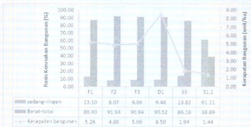
Gambar 3.3 Rasio kerusakan bangunan akibat gempabumi 27 Mei 2006 terhadap kerapatan bangunan pada tiap satuan bentuklahan di Kecamatan Pundong (Pengolahan data, 2012)
