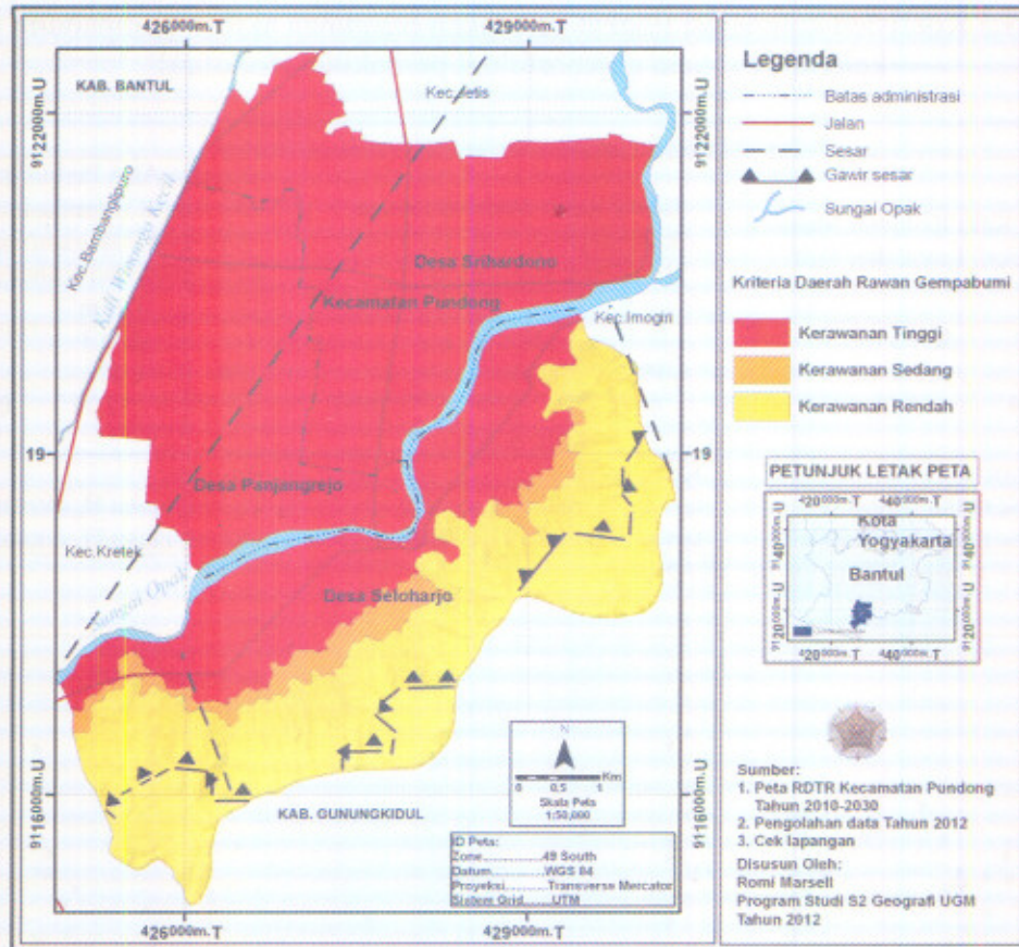
Gambar 3.5 Peta zona rawan gempabumi di Kecamatan Pundong berdasarkan pendekatan geomorfologi (Pengolahan data, 2012)
