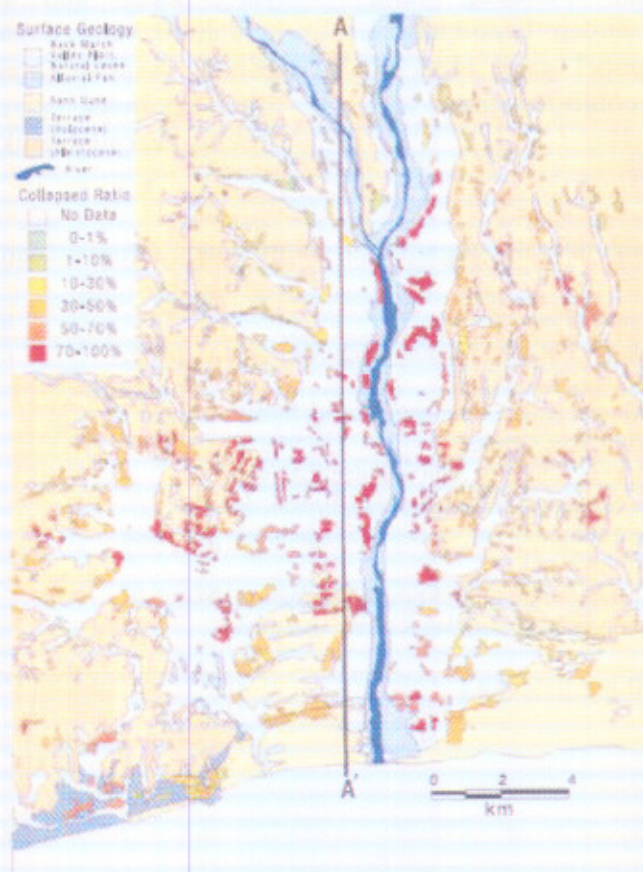
Gambar 1.3 Agihan kerusakan dan kondisi geomorfologi sepanjang Sungai Sagami ( Midorikawa , 2002)
