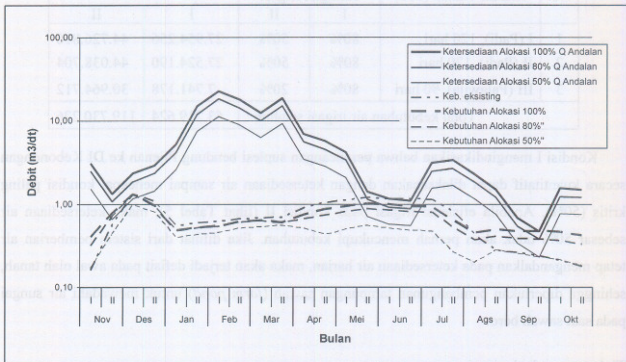
Gambar 3. Keseimbangan air di bendung Pijenan.
