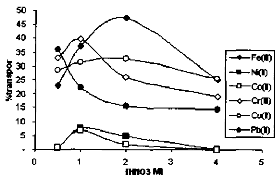
Gambar 4. Grafik hubungan konsentrasi pelucut terhadap persen transpor
