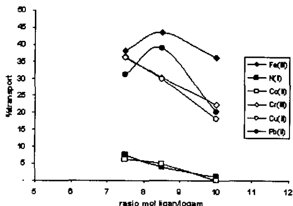
Gambar 3. Grafik hubungan persen transpor dengan rasio mol ligan : mol logam
