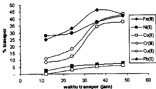
Gambar 5. Grafik hubungan waktu transpor terhadap persen transpor
