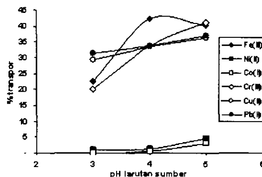
Gambar 2. Grafik hubungan pH larutan fasa sumber terhadap persen transpor
