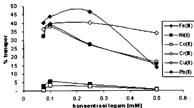
Gambar 6. Pengaruh konsentrasi logam terhadap persen transpor
