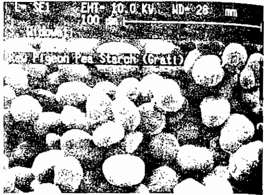
Gambar 2. Fotomikrograf granula pati gude varietas Grati
