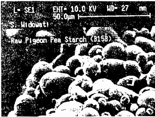
Gambar 1. Fotomikrograf granula pati gude varietas B15B
