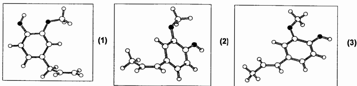
Gambar 2 Struktur perspektif eugenol (1), Cis-iseoeugenol (2) dan trans-iseoeugenol (3)
