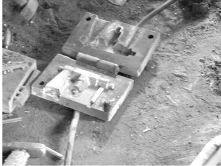
Gambar 5 Cetakan Permanen untuk Sambungan Pipa
