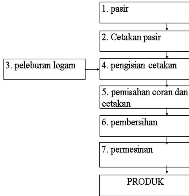
Gambar 17 Prosedur Pengecoran Kuningan di IKM Mitra
