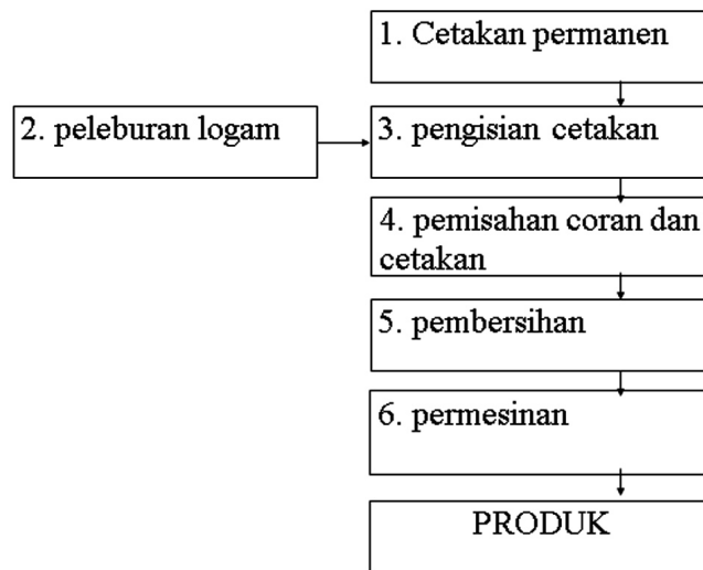
Gambar 18 Prosedur Pengecoran Kuningan yang Akan Diterapkan di IKM Mitra
