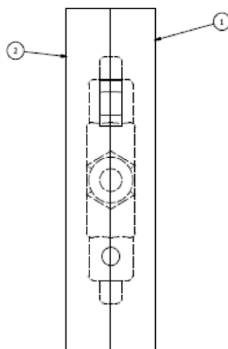
Gambar 1 Gambar Susunan Cetakan Permanen Sambungan T
