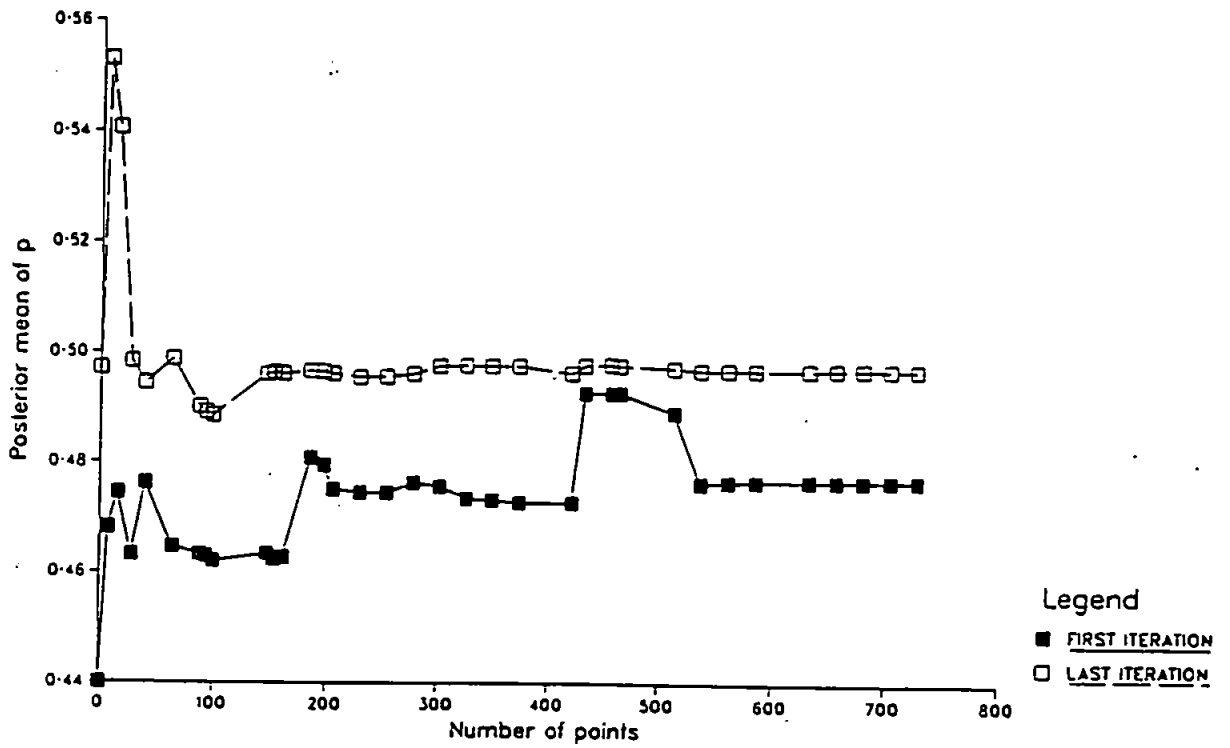
Convergence of posterior mean of p
