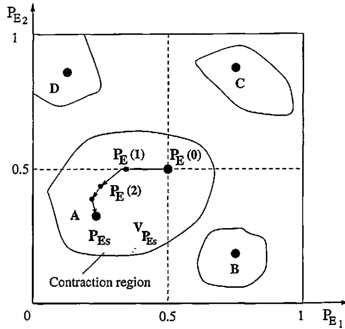
a) Convergent
