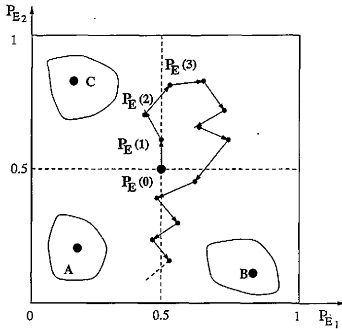
b) Nonconvergent
